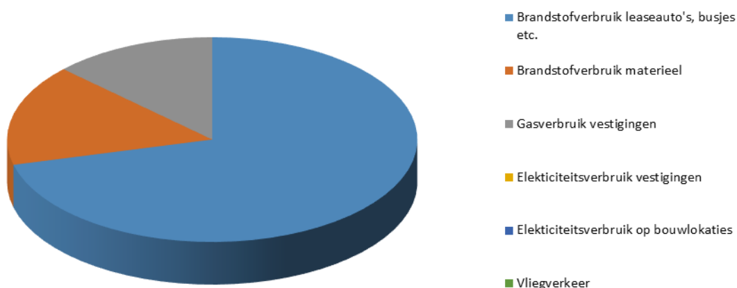
CO 2 -productie 2020 1e helft (verdeling in %)
