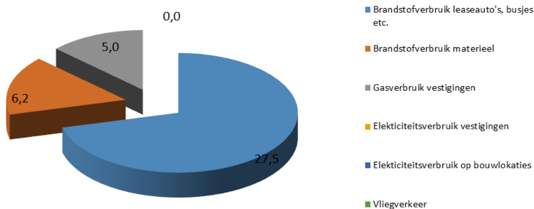
CO 2 -productie 2020 1e helft (ton/jaar)
